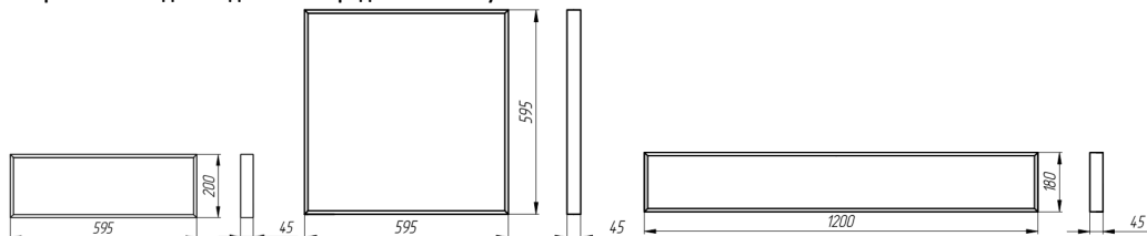
Рисунок 1 – Габаритные размеры светильников серии Офис IP54 (слева) и ЛПО IP54 (справа).
